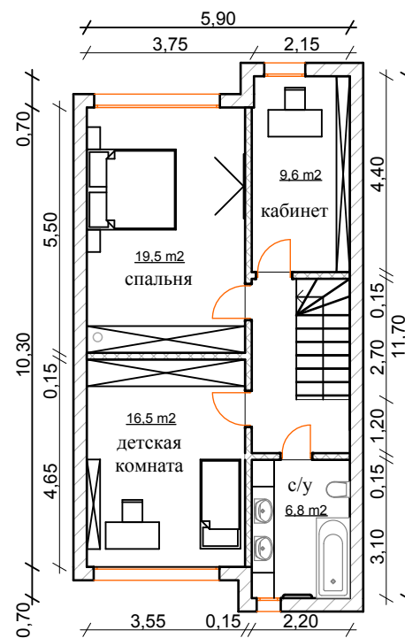
3 этаж 63,8 м 2
