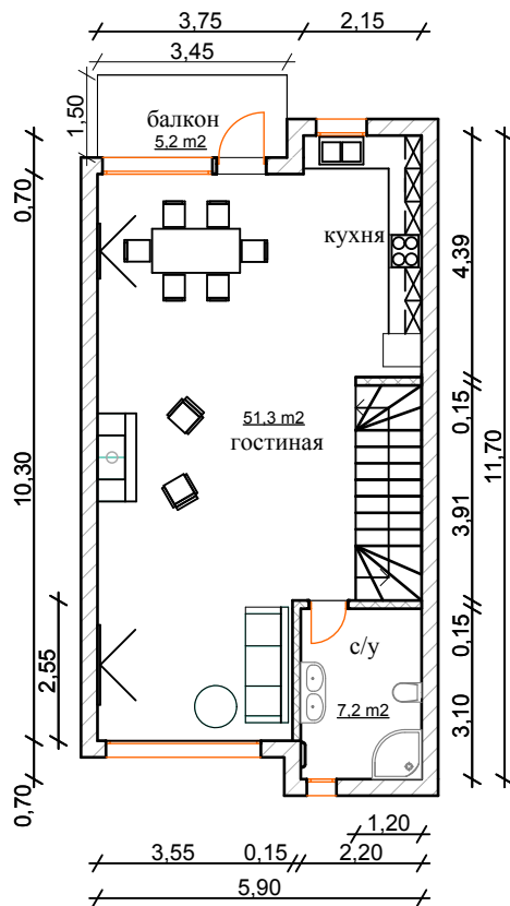
2 этаж 63,7 + 5,2 (балкон)=68,9 м 2
